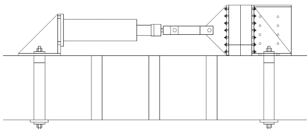
Figura 6: Montaje para fisuración
