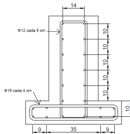
Figura 4: Armado de la probeta
