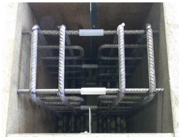
Figura 10: Vista interior de la probeta antes de hormigonar
