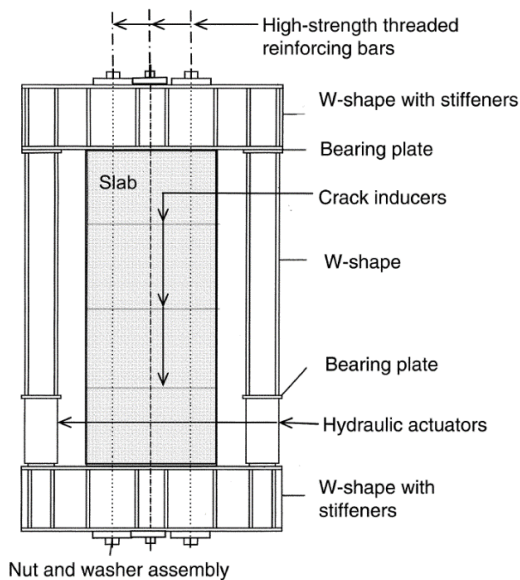
Figura 2: montaje propuesto por ACI 355.4-11 para fisuración
