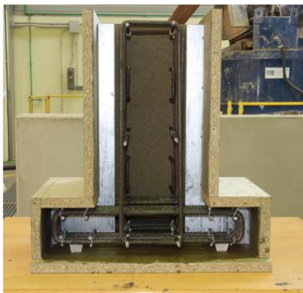
Figura 9: Probeta con armado sin tapa
