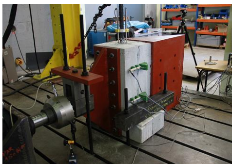
Figura 14: Montaje ensayo de tracción
