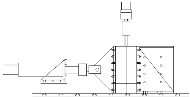
Figura 7: Setup ensayos de tracción
