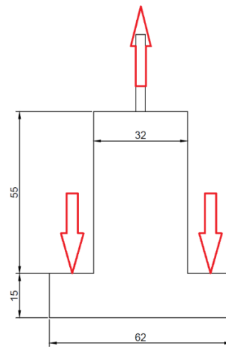
Figura 3: Nuevo diseño de probeta, cotas en cm
