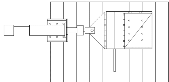
Figura 8: Montaje ensayo de cortante, vista en planta
