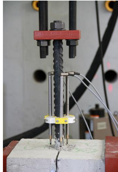
Figura 15: Instrumentación del anclaje
