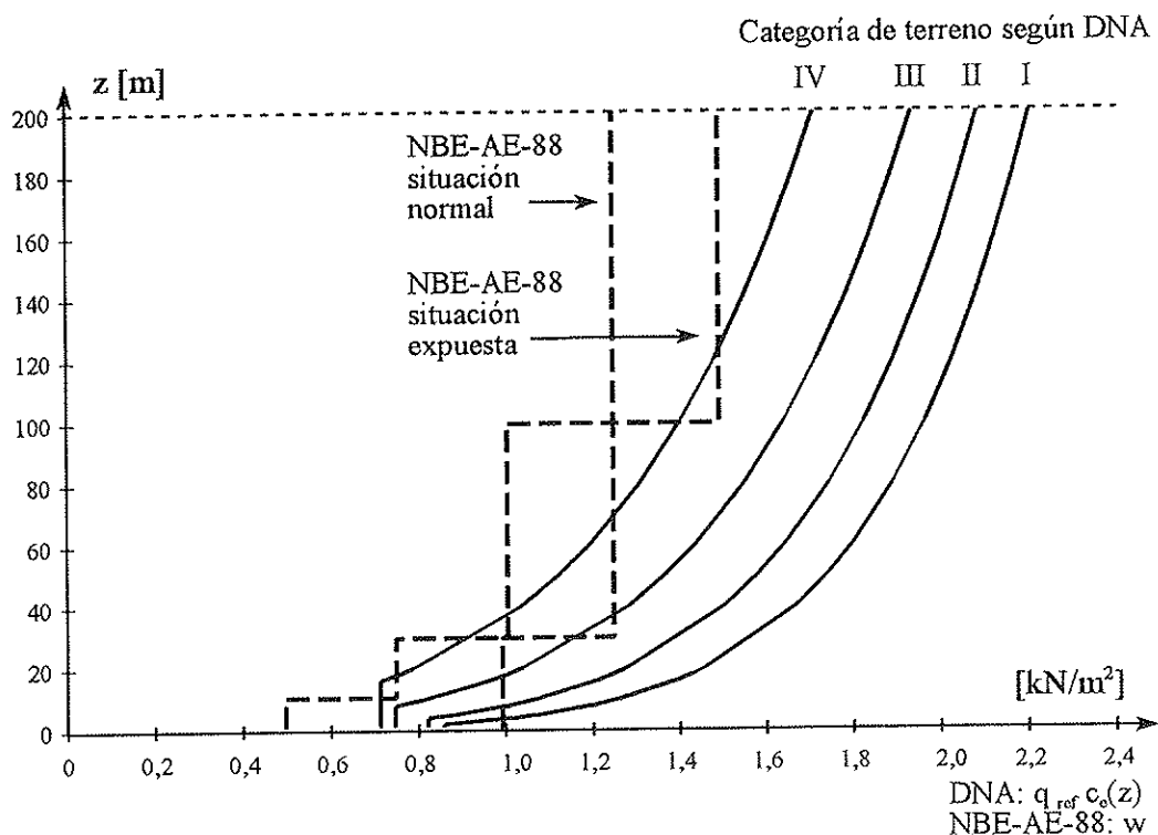
Figura 17. Comparación de la acción del viento según NBE-AE-88 [19] y DNA [4] en función de la categoría de terreno y de la altura sobre el suelo.
